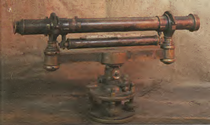
Meridianinstrument, som blev brugt til at opmåle Salt Lake dalen med.
